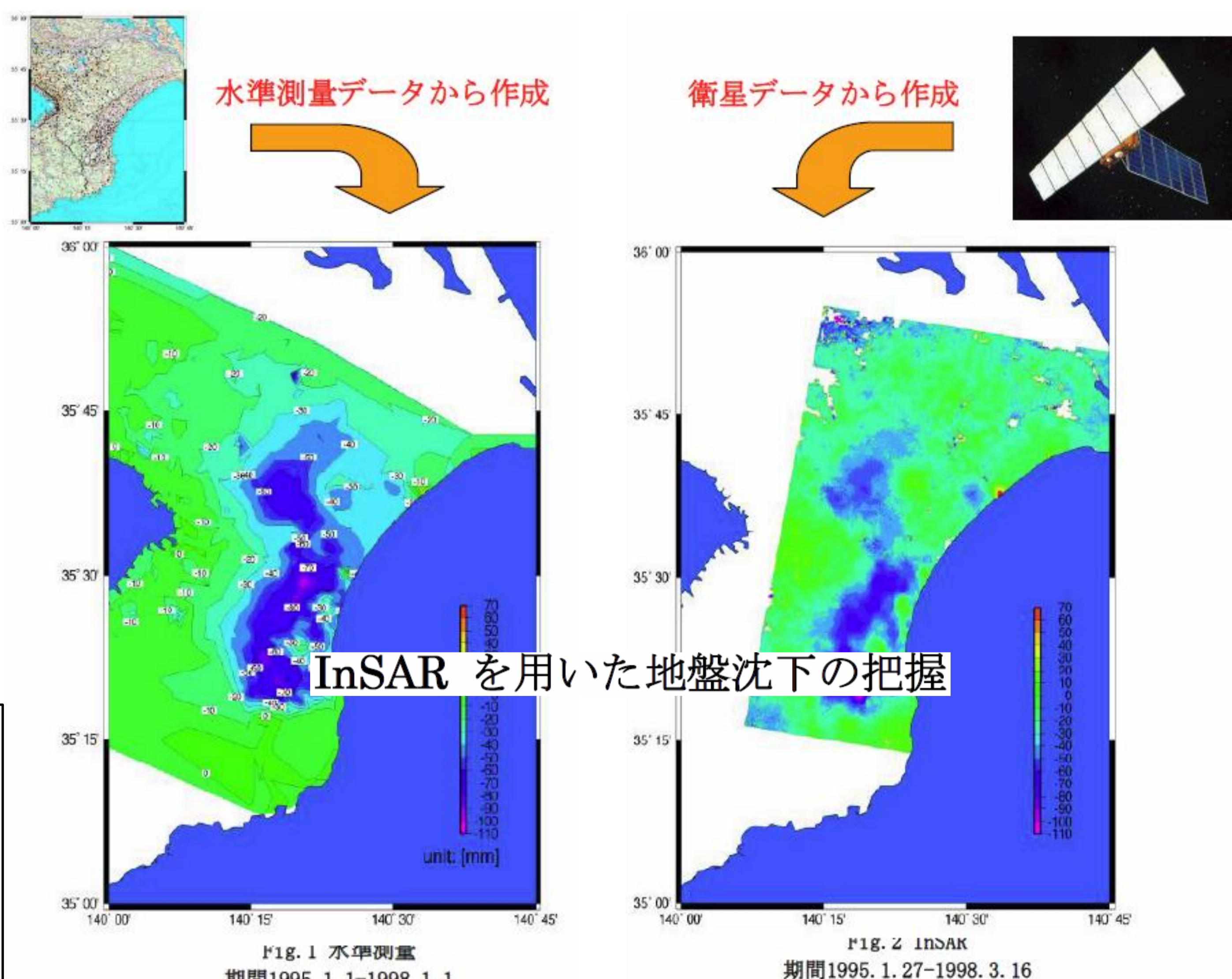
InSARを用いた地盤沈下の把握 提供：株式会社 NTTデータ CCS
