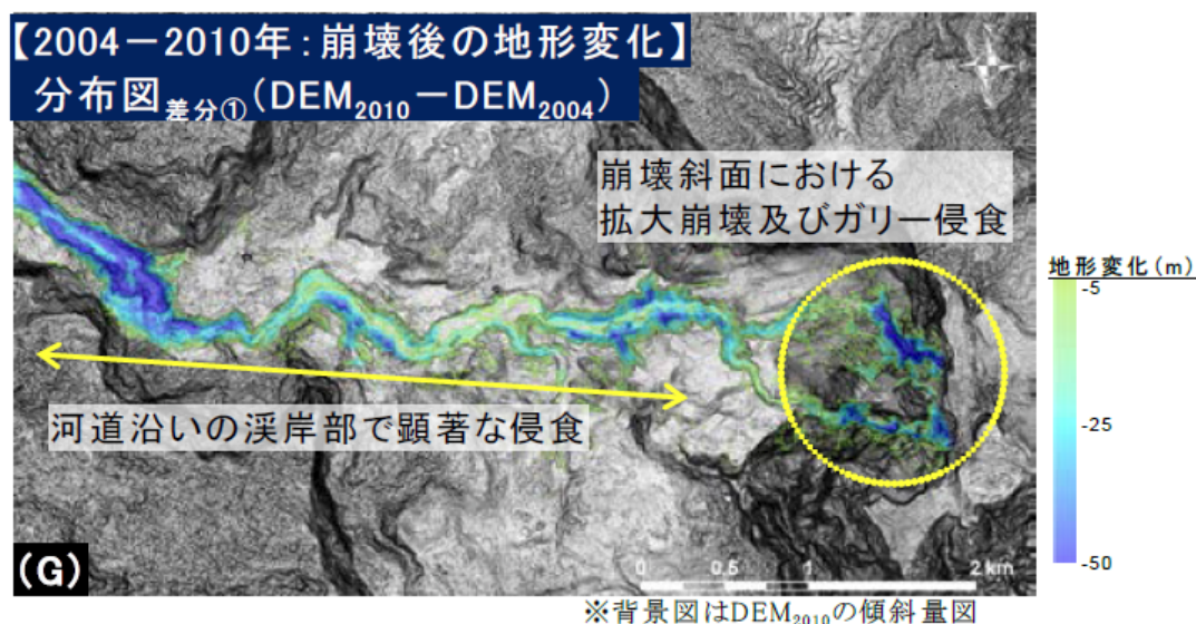
図-2.2.2 光学衛星画像より作成した DEM から抽出した崩壊地 5)
